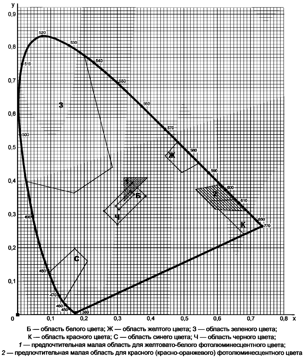
Рисунок Б.1 — Допустимые области цветности сигнальных и контрастных цветов фотолюминесцентных материалов на стандартном цветовом графике x, y МКО 1931 г.
