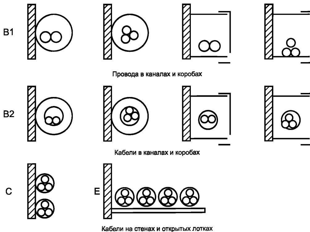
Рисунок С.1 — Методы укладки кабелей и проводов
