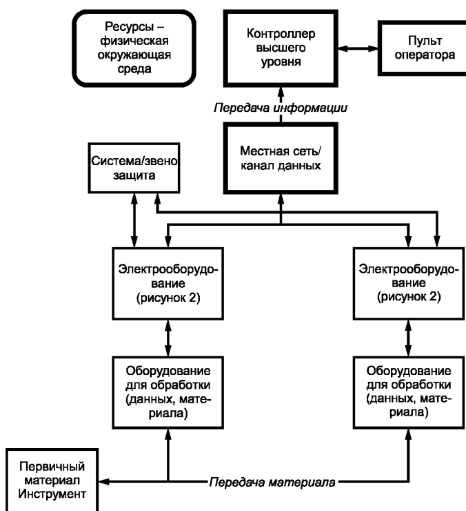
Рисунок 1 — Функциональная схема типовой производственной системы
